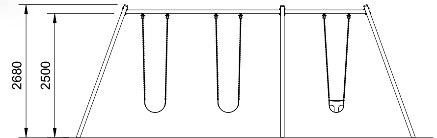
Elevation Scale: 1:75
