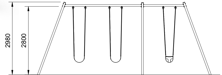
Elevation Scale: 1:75
