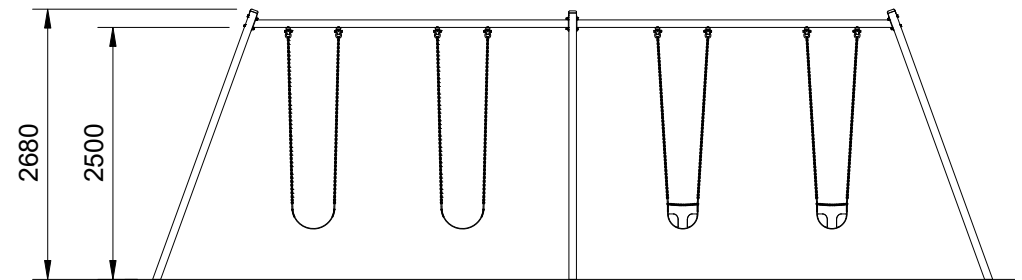
Elevation Scale: 1:75
