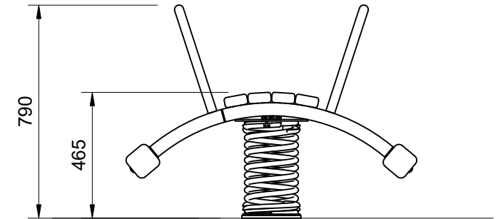
Elevation Scale: 1:20
