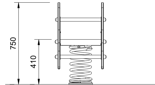
Elevation Scale: 1:20
