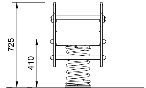
Elevation Scale: 1:20
