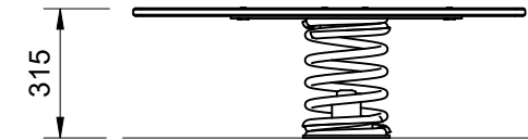
Elevation Scale: 1:20
