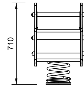
Elevation Scale: 1:20
