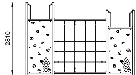
Elevation Scale: 1:70
