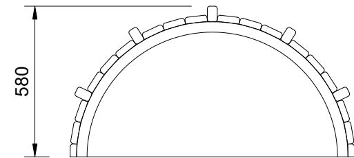
Elevation Scale: 1:20
