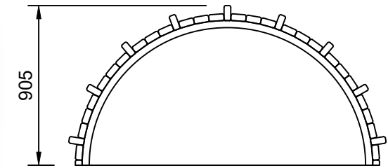
Elevation Scale: 1:30
