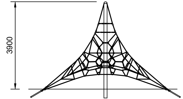
Elevation Scale: 1:100
