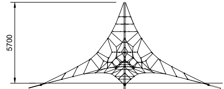
Elevation Scale: 1:150
