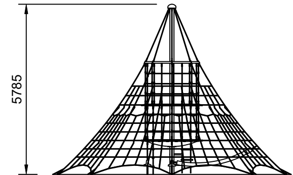
Elevation Scale: 1:130
