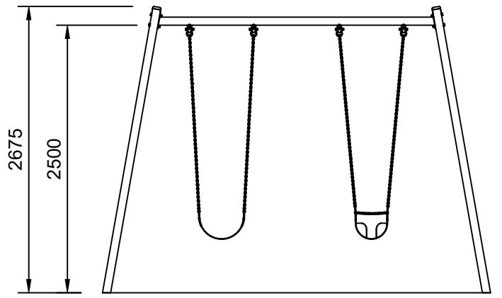
Elevation Scale: 1:50
