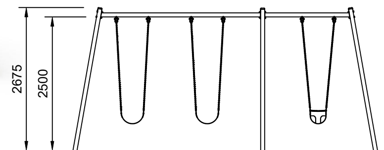
Elevation Scale: 1:70
