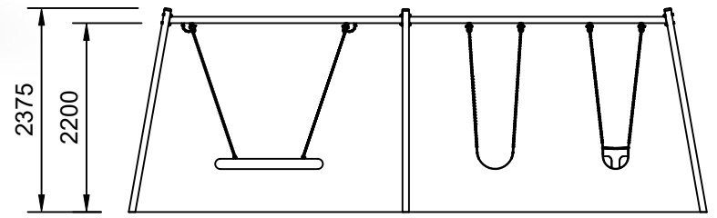
Elevation Scale: 1:80
