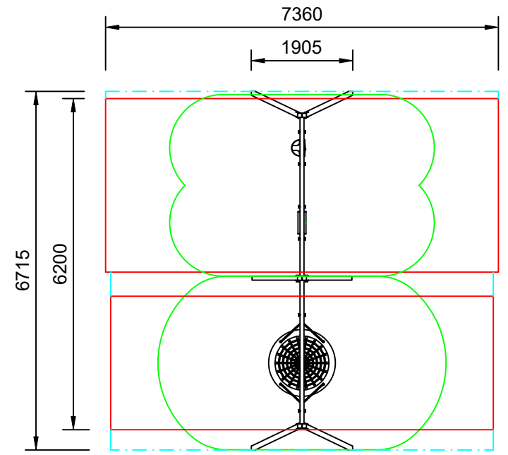
Plan View Scale: 1:100
