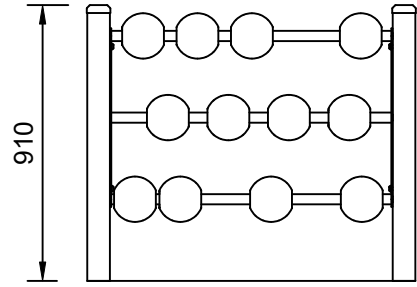
Elevation Scale: 1:25
