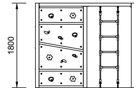
Elevation Scale: 1:50
