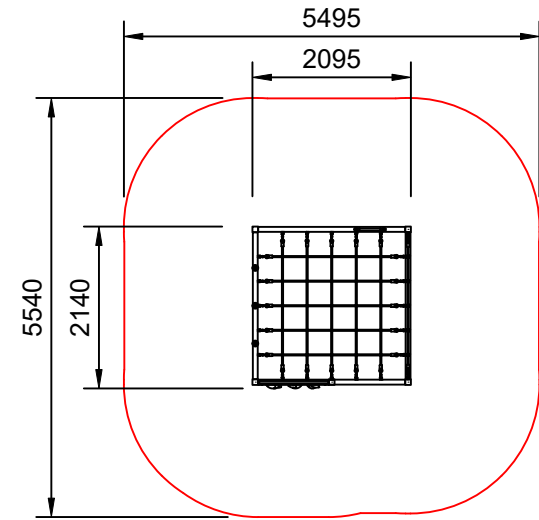
Plan View Scale: 1:100
