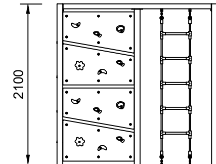
Elevation Scale: 1:50
