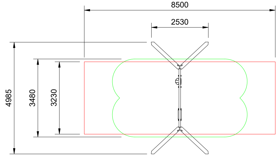
Plan View Scale: 1:100
