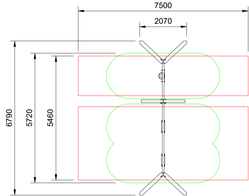
Plan View Scale: 1:100
