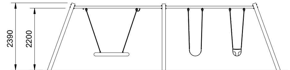
Elevation Scale: 1:80
