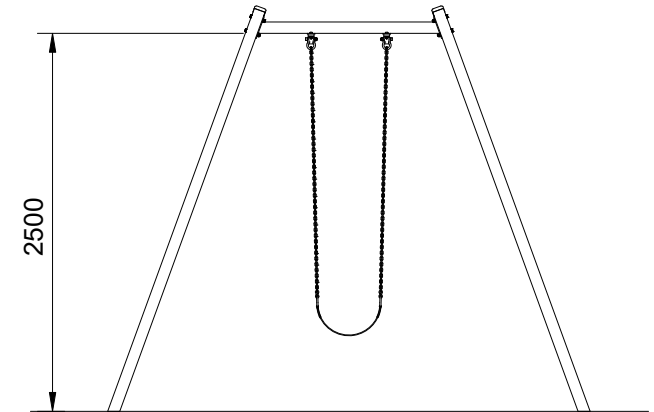
Elevation Scale: 1:50
