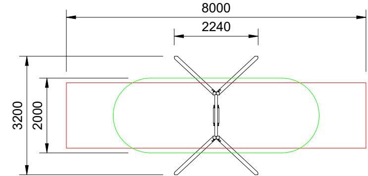
Plan View Scale: 1:100
