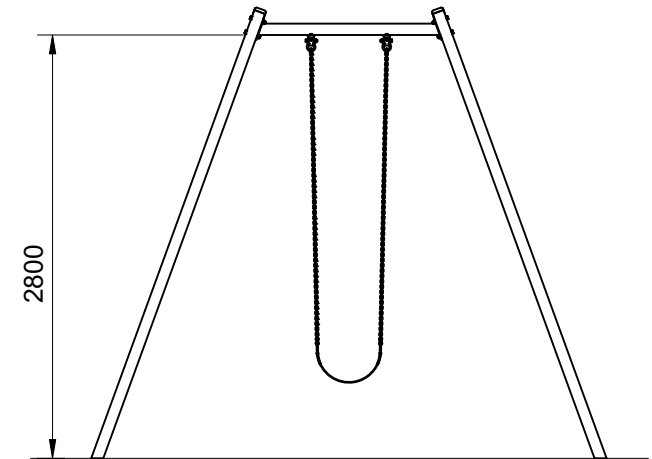
Elevation Scale: 1:50
